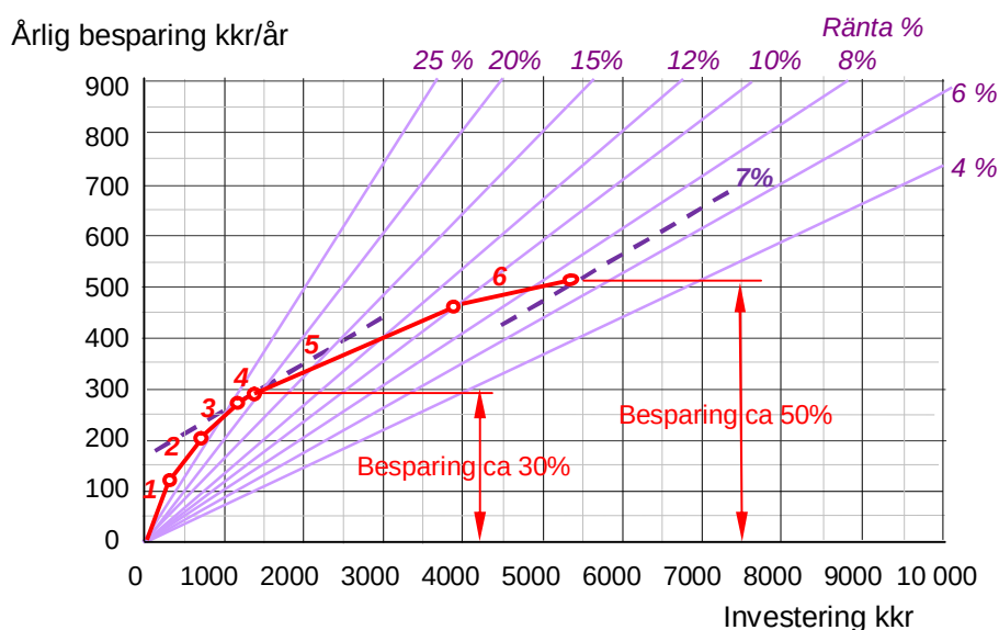
Figur 1.2 Åtgärdspaketet i internräntediagram. Diagrammet visar den faktiska avkastningen, som en investering ger, räknad i reallräntemått. Genom att kombinera åtgärder i ett paket, där de lönsammaste delarna bidrar till delar som på egen hand hade varit olönsamma, kan energibesparingen ökas till upp mot 50 %.
