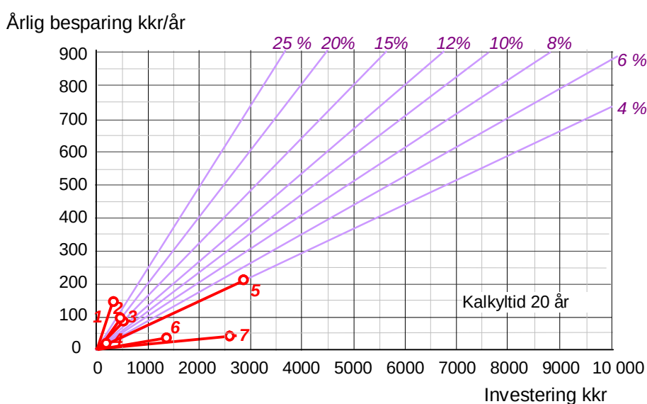
Figur 2.13 Åtgärdernas lönsamhet presenterad i ett internräntediagram. Procentsatserna anger internräntan. Råda punkter med linjer till origo representerar olika åtgärder. Diagrammet gäller för kalkyltiden 20 år.
