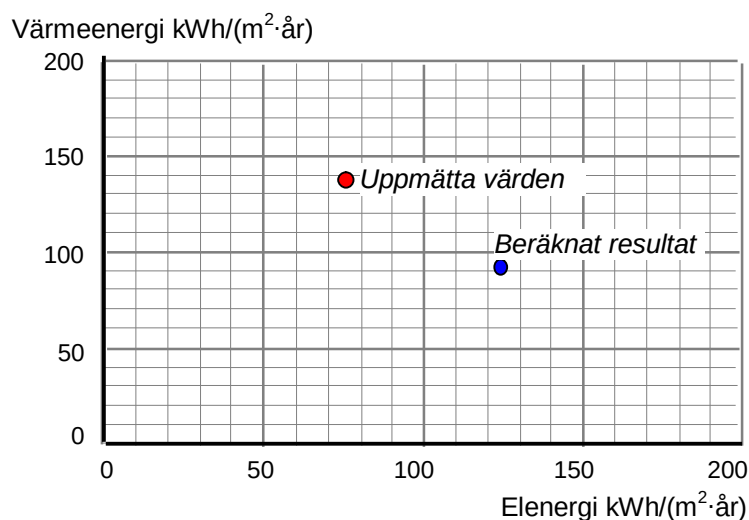
Figur 6.3 Jämförelse av resultaten av den första energiberäkningen med den uppmätta verkliga energianvändningen.
