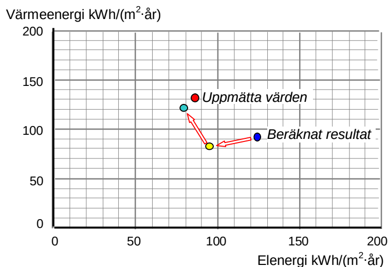
Figur 6.4 Jämförelse av resultaten av energiberäkningar med uppmätt energianvändning efter justering av osäker indata.
