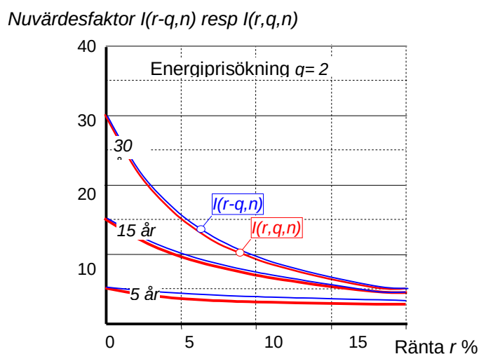
Figur 2.10 Approximeringen I(r-q,n) och det matematiska värdet I(r,q,n)
