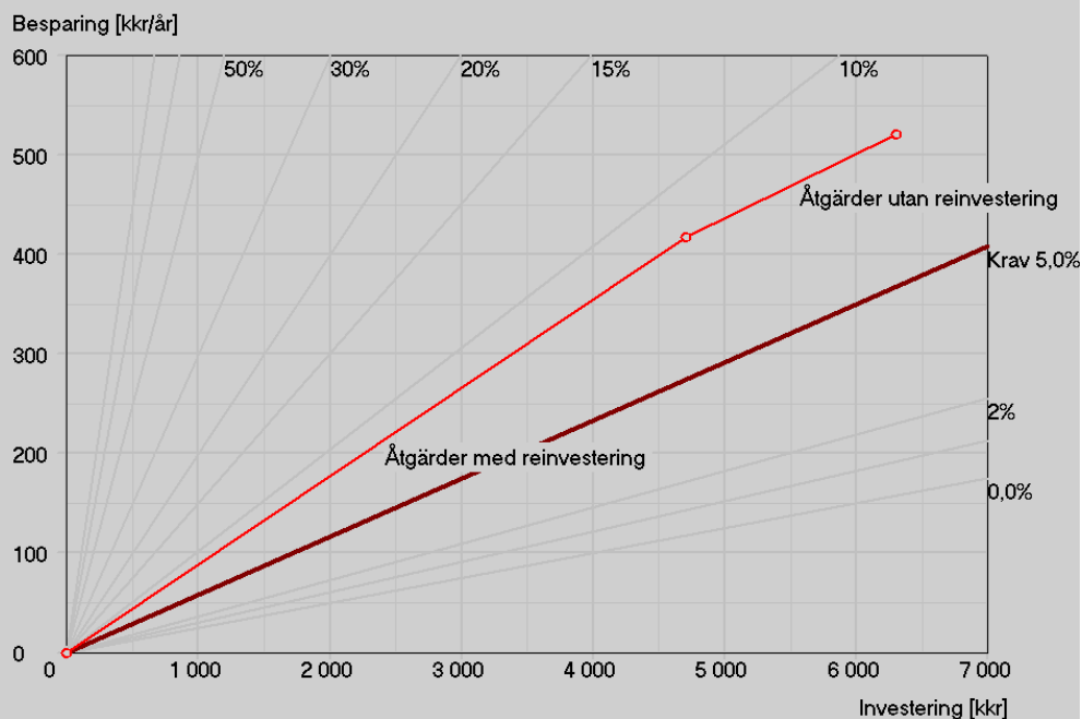
Figur 2.18 Åtgärds paketet enligt tabell 2.2 med reinvestering.
