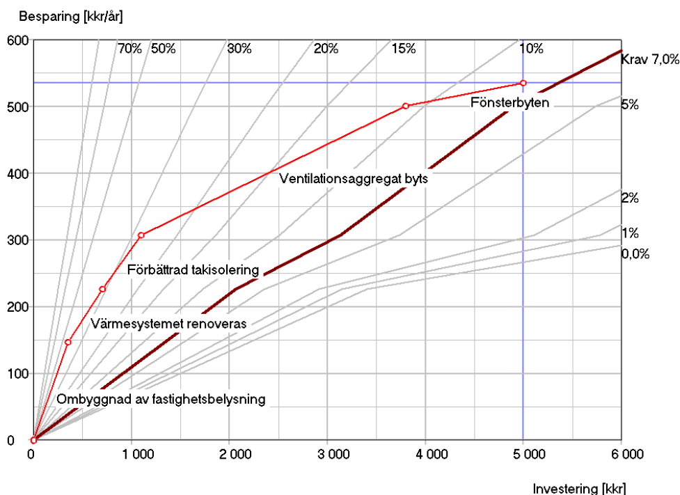
Figur 6.6. Exempel på bildning av åtgärdspaket presenterad i ett internräntediagram med hjälp av Totalverket . Beställarens lönsamhetskrav är 7 % och den bedömda framtida energiprishöjningen 2 % utöver inflationen. Det innebär att beställarens lönsamhetskrav är att åtgärdspaketet skall ge högre real avkastning än 7 - 2 = 5 %.
