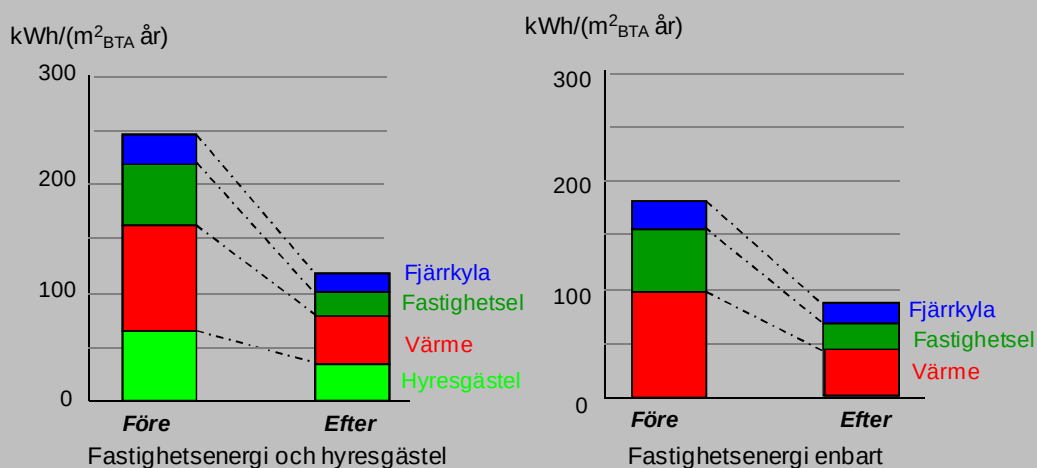
Figur 11.1 Uppmätt energianvändning efter genomföring åtgärds paket. Diagrammen vänster visar resultatet med hyresgästel och höger bild visar resultatet utan hyresgästel.
